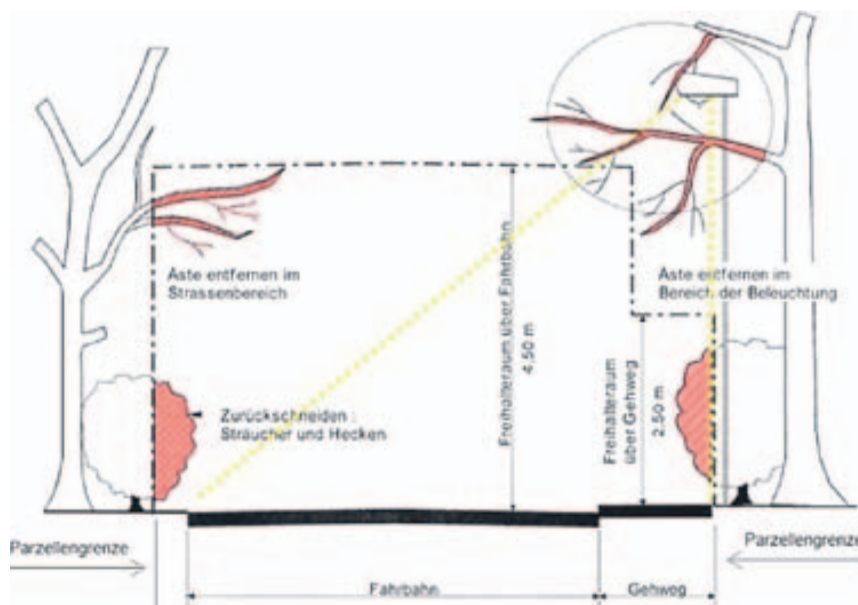
Freizuhaltenes Lichtraumprofil gegenüber Strassenraum
